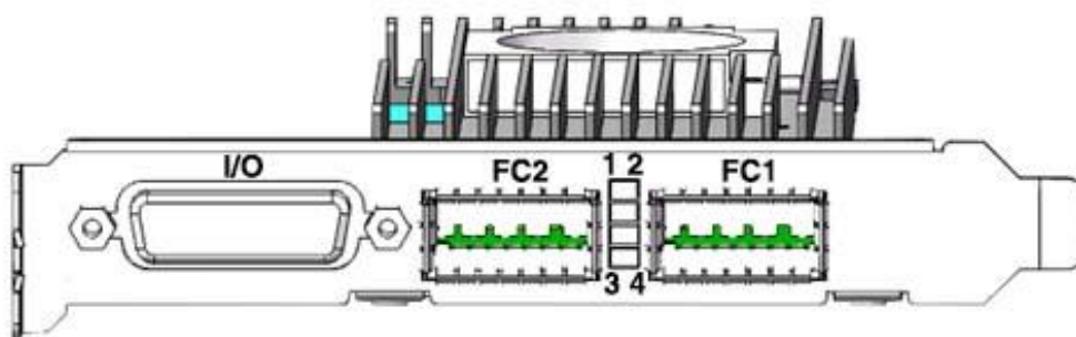
图 6 前面板示意图
