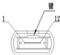
图 8 光模块 MPO 插座点位图
