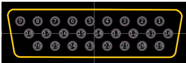
图 9 前面板 D-SUB_HR26_FEMALE 接口点位图
