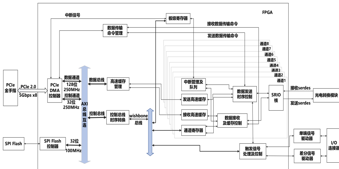
图 2 原理框图
